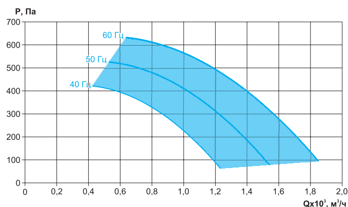
ВРС-К-50-30/22-РЦ-0,55/3000/220-380
